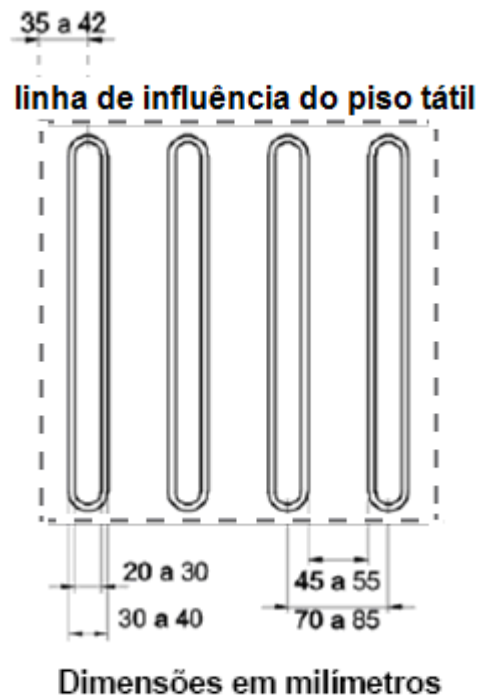
Fig.02 – Planta - Modulação do piso tátil direcional
