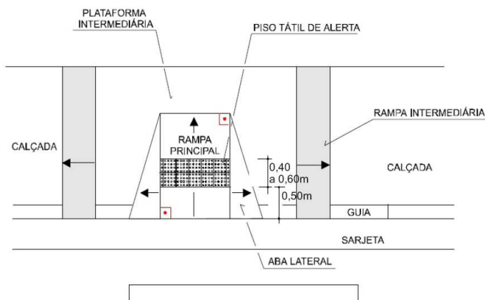
Fig.05b – Planta - Rebaixamento TIPO II Piso tátil no acesso principal.
