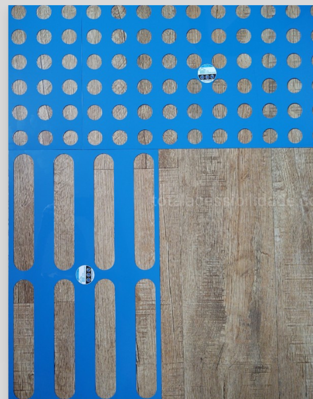
FOTO ILUSTRATIVA DO GABARITO DE FIXAÇÃO DE PISOS DISCREET TOTAL ACESSIBILIDADE
