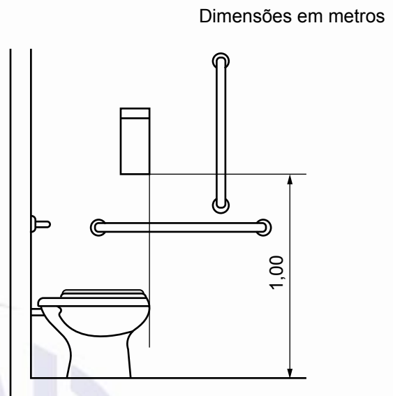
Figura 126 – Localização da papeleira de sobrepor (interfolhado) – Vista lateral
